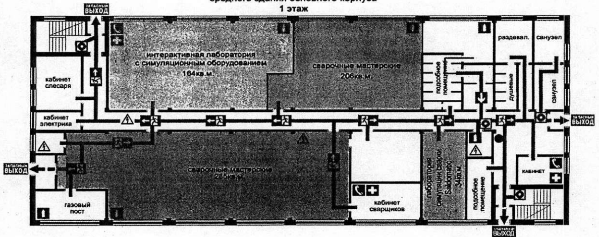
План среднего здания основного корпуса 1 этаж
