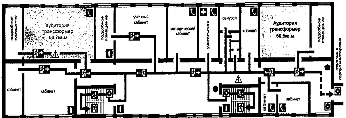
План учебного здания основного корпуса 2 этаж
